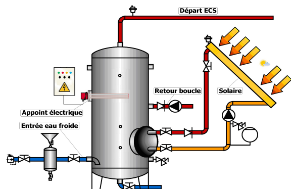
EAU CHAUDE SOLAIRE + APPOINT ELECTRIQUE
