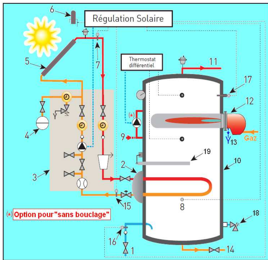
⇒ Schéma -4 : RECHAUFFEUR SOLAIRE associé au HYDROGAZ (appoint)
