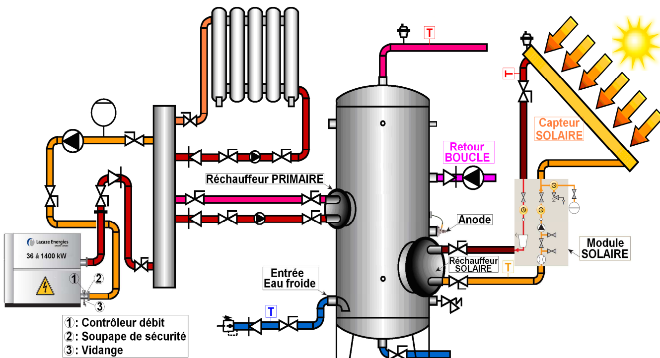
⇒ Schéma -3 : RECHAUFFEURS SOLAIRE & PRIMAIRE
