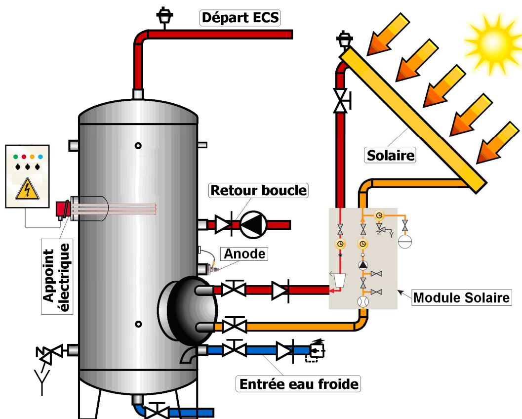
⇒ Schéma -2 : Ballon tampon solaire + Echangeur interne (réchauffeur Solaire)/Electrique
