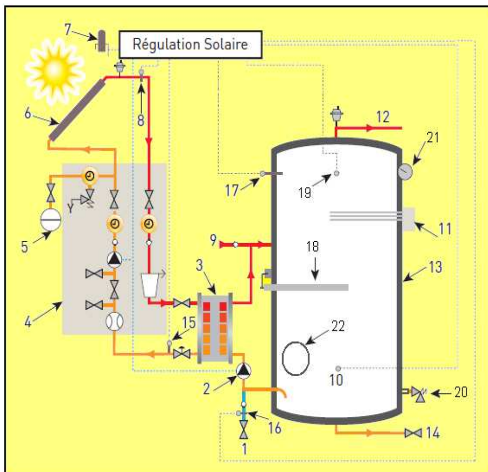
⇒ Schéma -1 : Ballon tampon Solaire + Echangeur extérieur /Electrique
