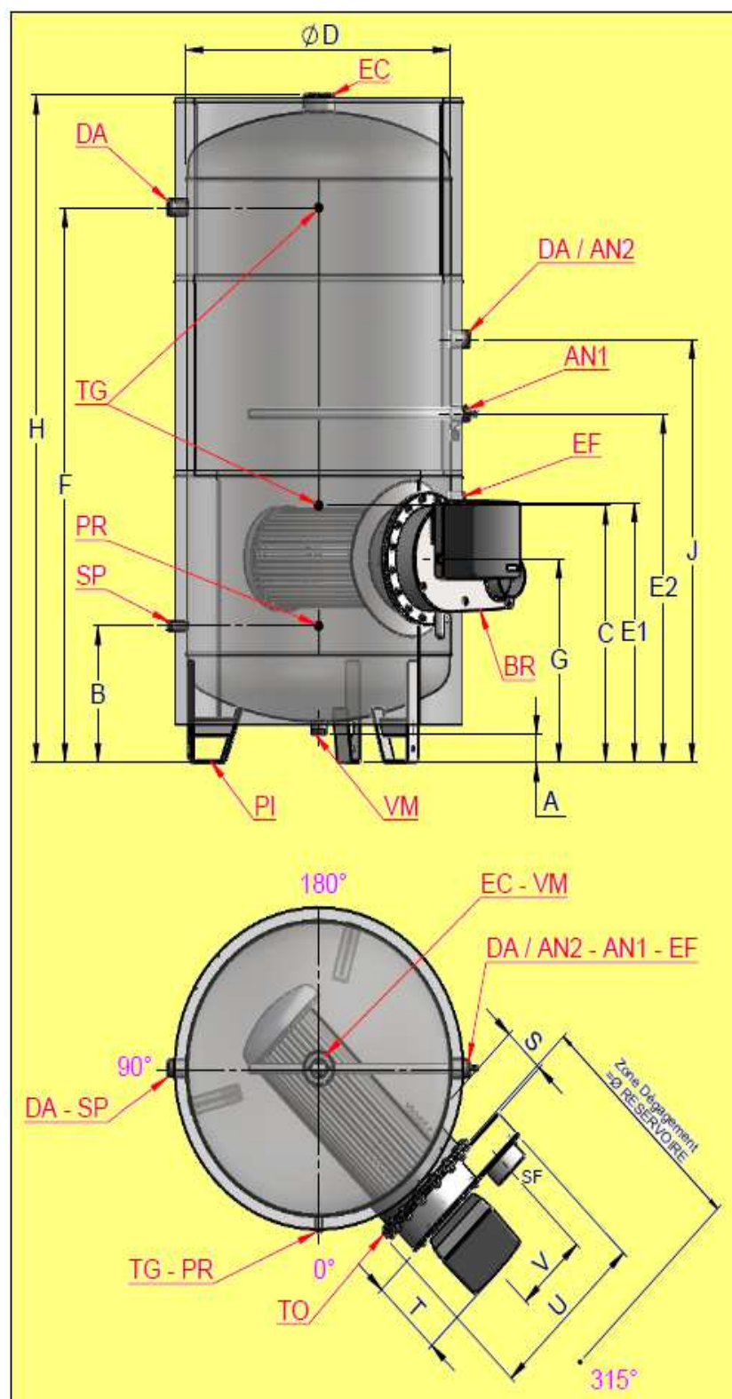
Plan indicatif des Réservoirs 750 à 6 000 l (Gamme PREFERENCE)
