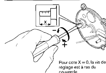
Réglage du déflecteur (cote X)
