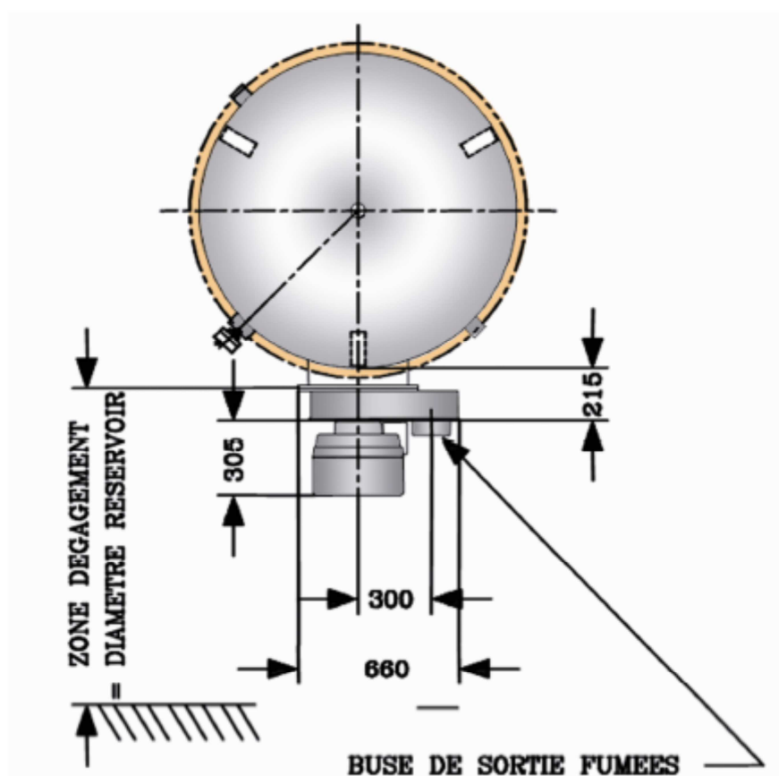
Figure N°3123.12 : Figure indicatif d'encombrement Brûleur / Echangeur
